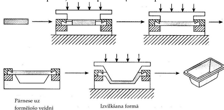
7.6. attēls. Cietā stāvokļa veidošana ar izvilšanu.
