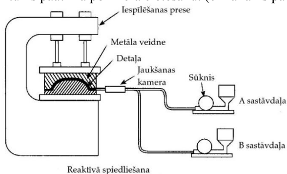
7.16. attēls. Reaktīvās spiedienliešanas shēma.
