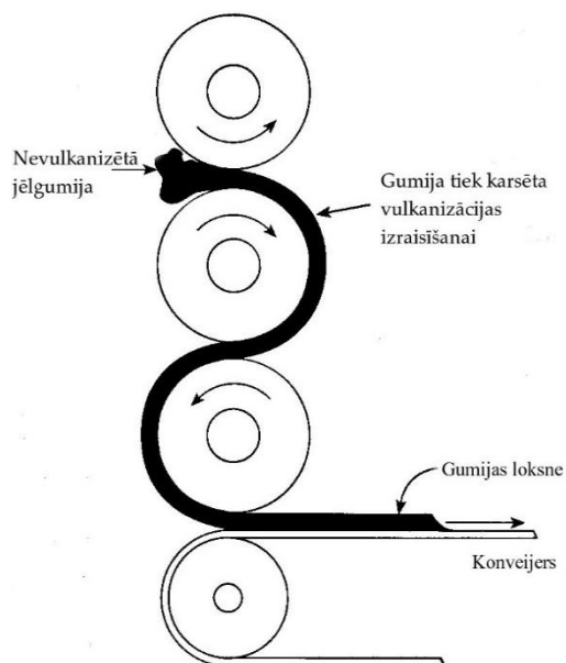
7.4.attēls. Kalandrēšana
