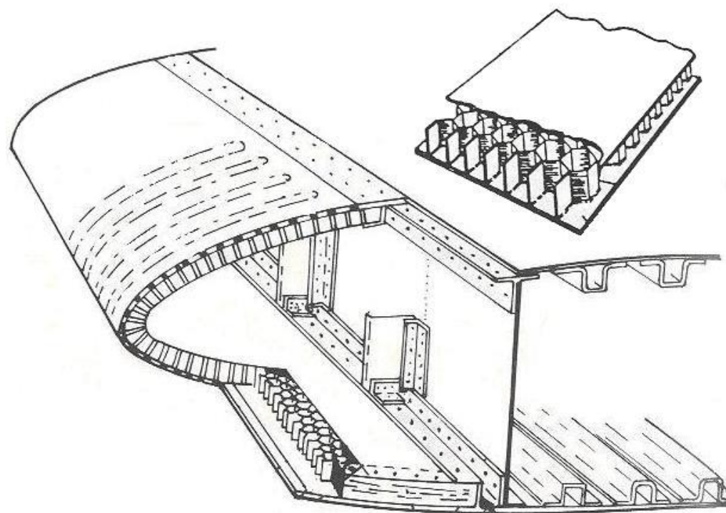
9.4. attēls. Sendviča tipa lidmašīnas spārnu konstrukcija.
