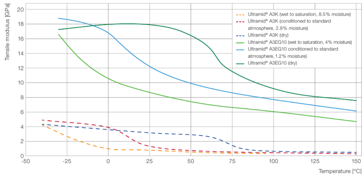
4.4. attēls. Stiepes modulis Ultramid ® A3K un A3Eg 10 atkarībā no temperatūras un mitruma.
