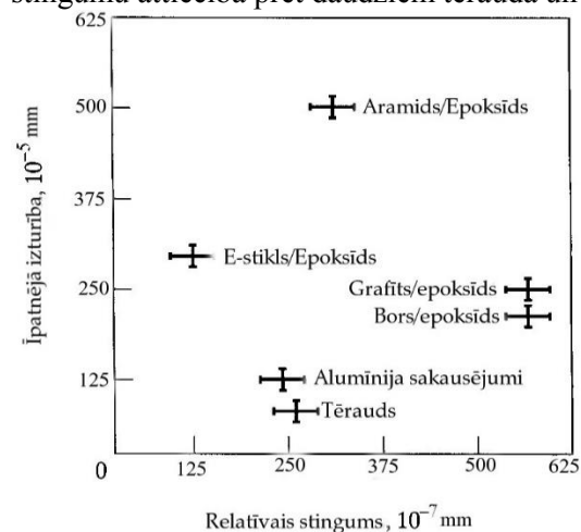
7.24. attēls. Īpatnējā izturība un relatīvais stingums dažiem epoksīda matricas polimēriem.
