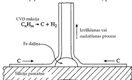
3.4. attēls. Oglekļa nanocaurulītes audzēšanas mehānisms katalītiskā CVD procesā.
