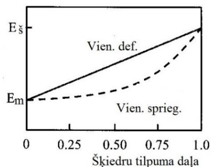
4.2. attēls. Kompozīta elastības modulis pie vienādu deformāciju un vienādu spriegumu nosacījumiem. Līknes iegūtas no iepriekš izveidotajiem vienādojumiem.
