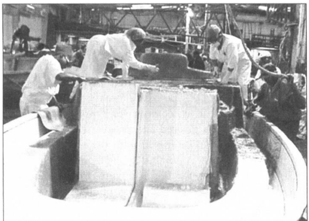
5.4. attēls. Ar stikla šķiedrām armētu sveķu izlīdzināšana laivas izgatavošanā.
