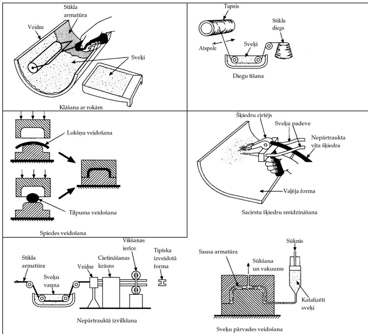
8.2. attēls. Ar šķiedrām armētu kompozītu ražošanas metodes.
