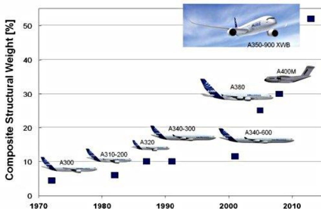
9.8. attēls. Kompozīto materiālu izmantošana lidmašīnu tehnoloģijā.
