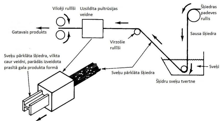
5.6. attēls. Izstiepšanas (pultrūšijas) metode kompozītu ražošanas procesā.
